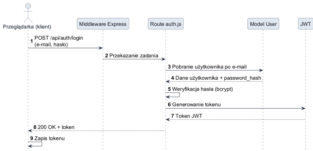
Rys. 3. Diagram sekwencji – logowanie użytkownika
