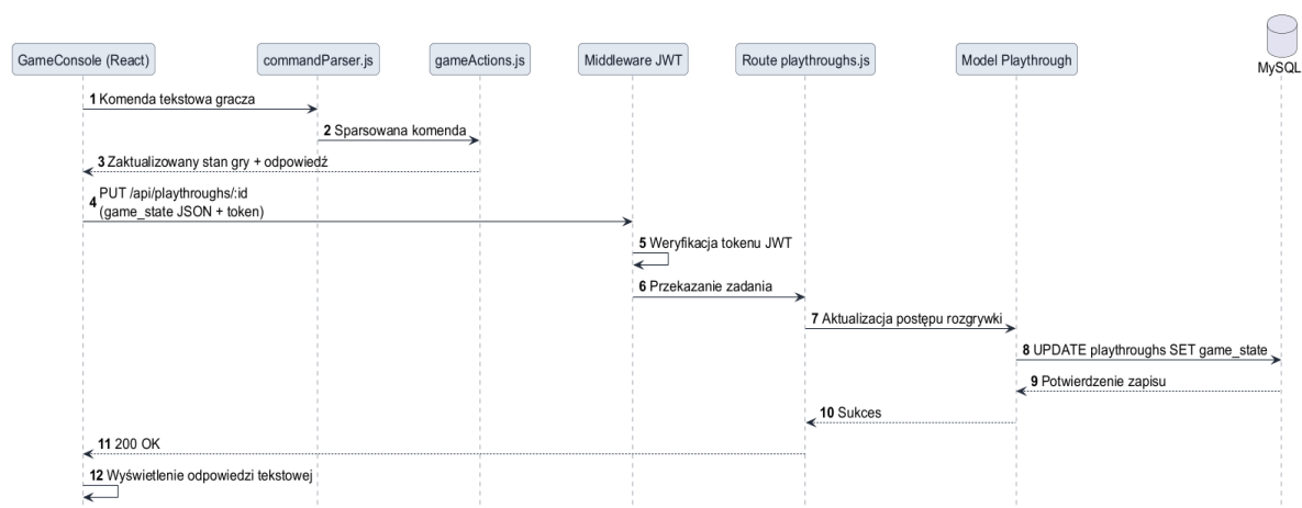
Rys. 5. Diagram sekwencji – krok rozgrywki
