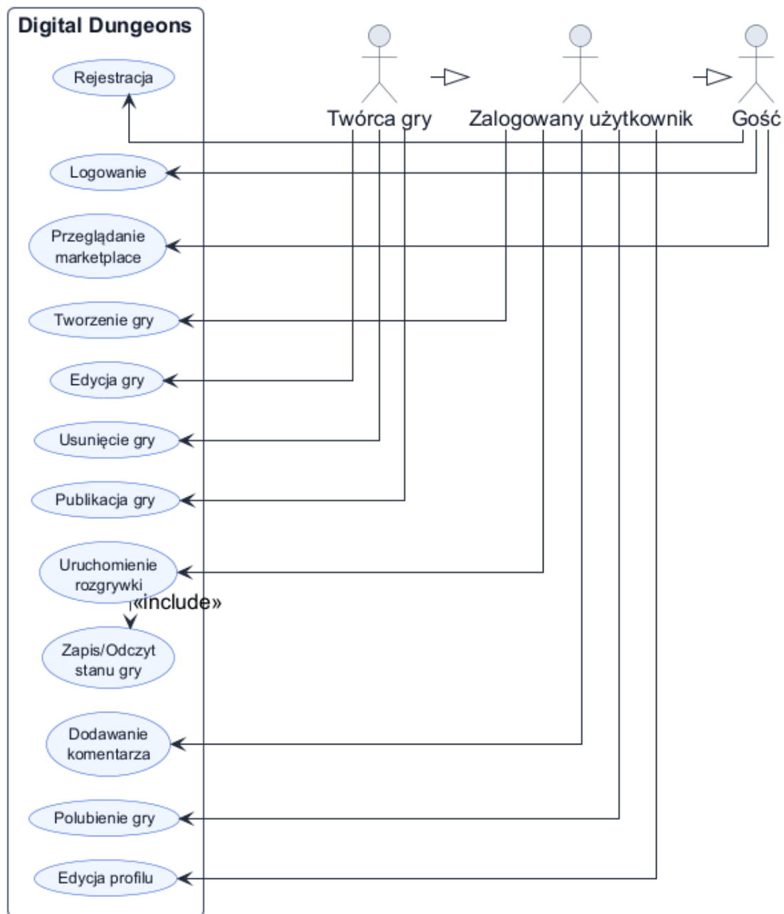
Rys. 2. Diagram przypadków użycia
