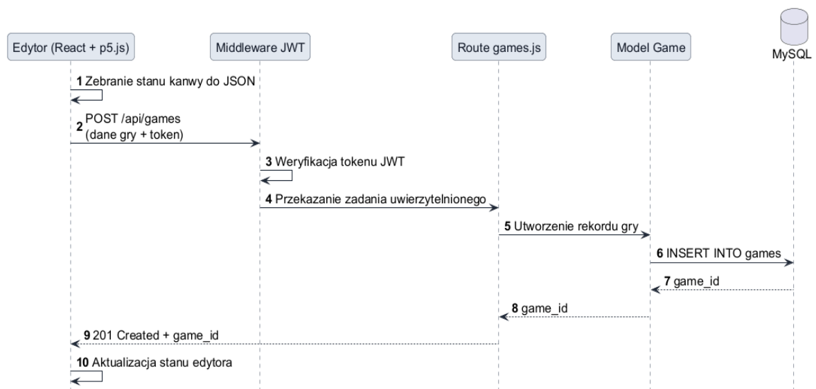
Rys. 4. Diagram sekwencji – zapis gry przez edytor
